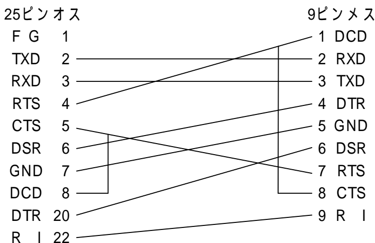
Dsub25ピンオス - Dsub9ピンメス 1.5mクロスケーブル結線図
