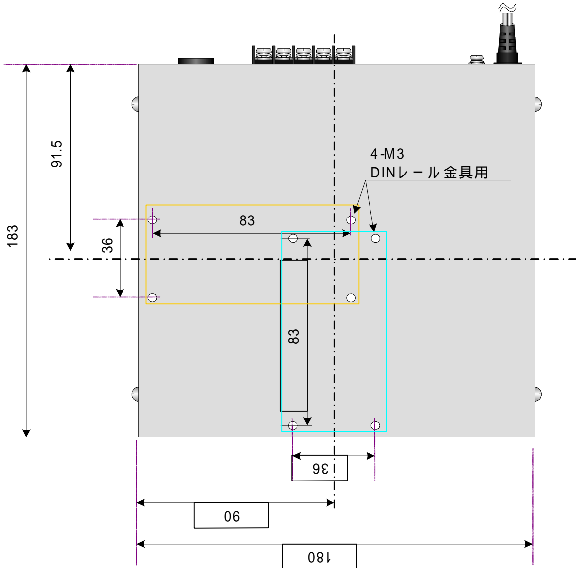
【 Enet-485/ AC DINレール取付金具穴位置寸法図】
